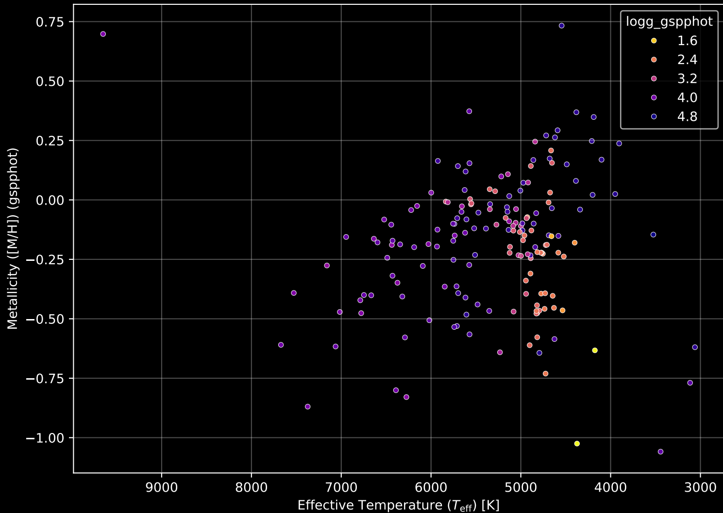
APOGEE DR17 Field: [CVZTILE_106+33_btx] Stellar Population Parameters (n= 173)
